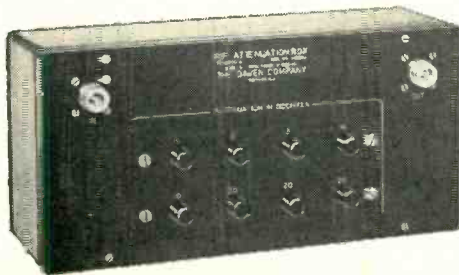
RF ATTENUATION BOX TYPE 650
